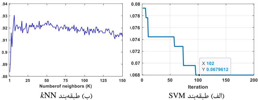
نمودار (۷) عملکرد طبقه‌بندی‌های مختلف با استفاده از چهار شاخص
