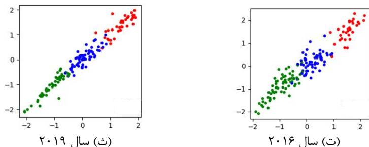
شکل (۳) نتایج خوشه‌بندی با استفاده از الگوریتم FDC
